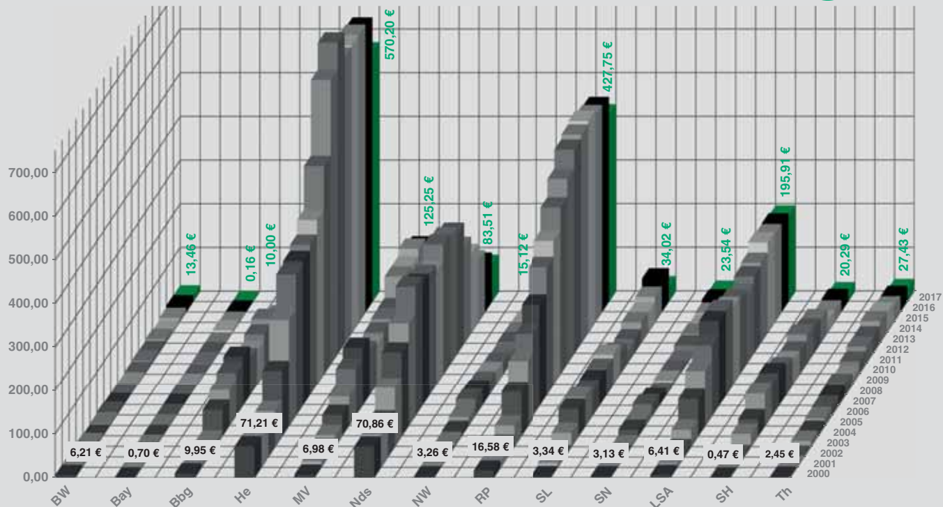
Abb. 3: Kassenkreditbestand der Landkreise in Euro pro Kopf nach Ländern: 2000-2017
